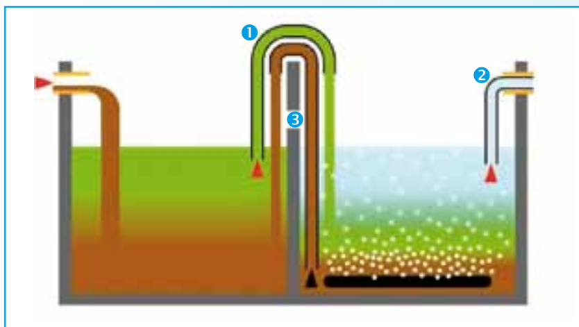
Schematische Darstellung der Funktionsweise einer SBR-Anlage
